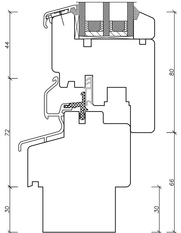
3-GLASS U_g = 0,7
